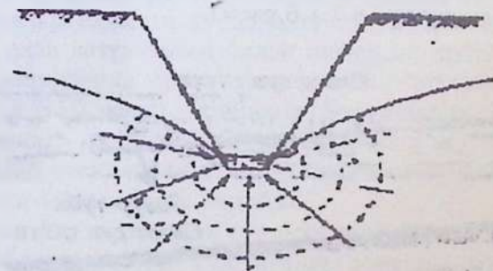
8.7.1.5-расм. Сизот сувнинг зовурга томон оқиб бериш тизими: 1-тенг босимли чизиқлар (эквипотен цикллари); 2-сув оқими чизиқлари.
