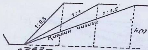
8.7.1.3-расм. Қиялик катталиги. h -зовур чуқурлиги.
