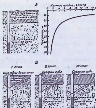
8.7.4.3-расм. Тик зовурнинг таъсир тизими:
