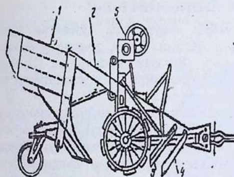
8.7.2.1-расм. КМ-800 маркали канавокопатель 1 - ишчи органи 2 - рамаси, 3 - кескиш органлари, 4-растегич
