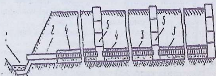
8.7.3.4-расм. Ёпиқ зовурнинг бўйлама қирқими:
