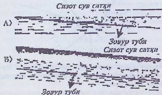
8.7.1.6-расм. Сизот сув оқимида кўндаланг (а) ва бўйлама (б) зовурларнинг иш тизимлари.
