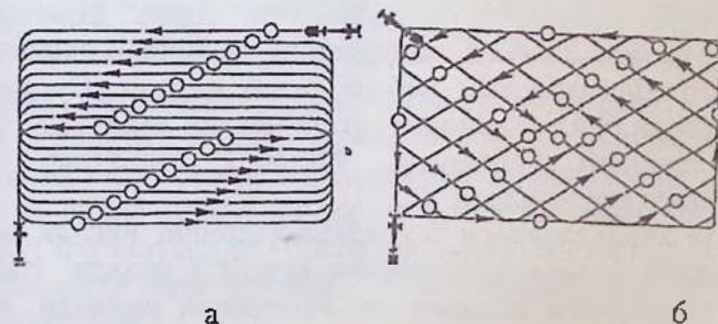
8.5.2.8-расм. Ерни жорий текислаш тартиби: а-бўлакларга ажратиб далани узунасига ёки кўндалангига текислаш, б-далани диагональ бўйича текислаш.
