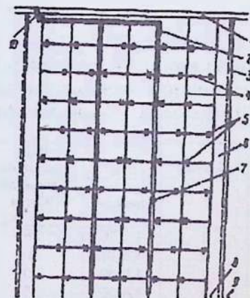
9.3.2-расм. Муваққат зовурлар ва чекларни жойлаштириш:
