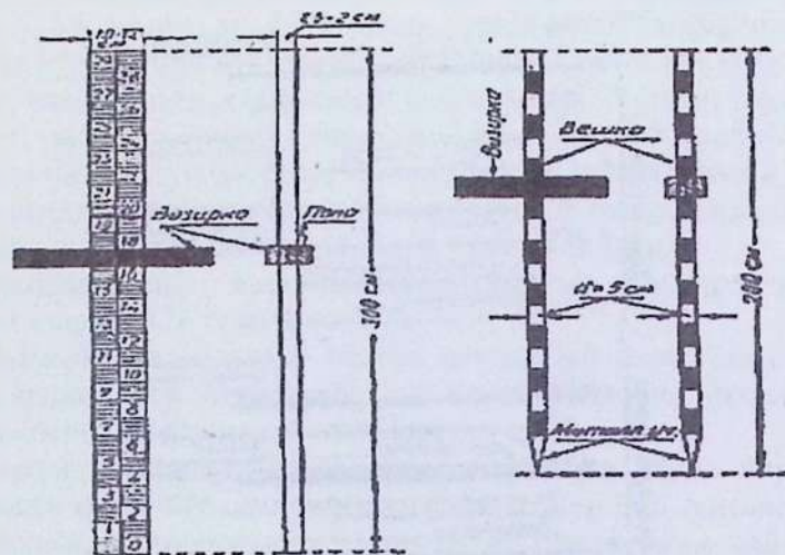
8.5.2.4-расм. Текислаш ишларини бажаришда қўлланиладиган рейка - визиркалар.
