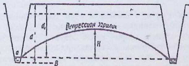
8.7.1.4-расм. Зовурнинг сизот сувларига таъсири:
