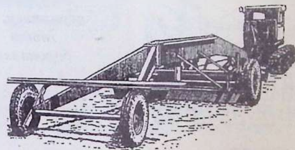
ПА-3 маркали узун базали текислагич
