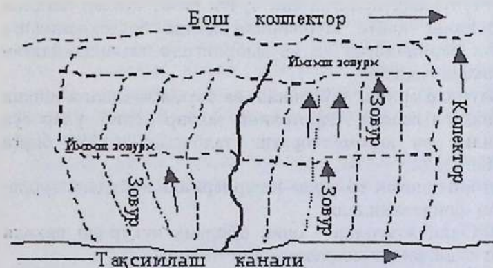
7.1.1-расм. Очiq зовур ва коллекторлар тизими.
