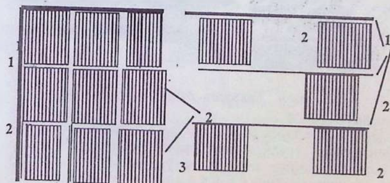
8.6.4.1-расм. Эгатлаб шўр ювишда бўйлама (а) ва кўндаланг (б) ўқариқларни жойлаштириш тизими.
