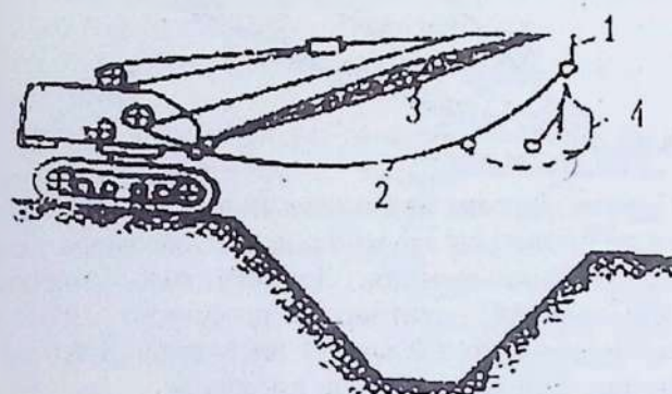
8.7.1.2-расм. Очiq зовур. 1 ва 2-кўтариш ва тортиш пўлат арқони; 3-стреласи; 4-ковуши.
