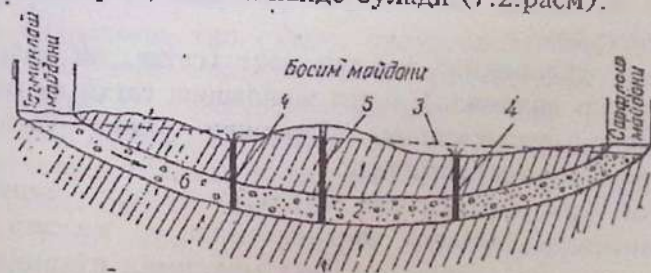
7.2-расм. Босимли сув ҳовузининг тузилиши.
